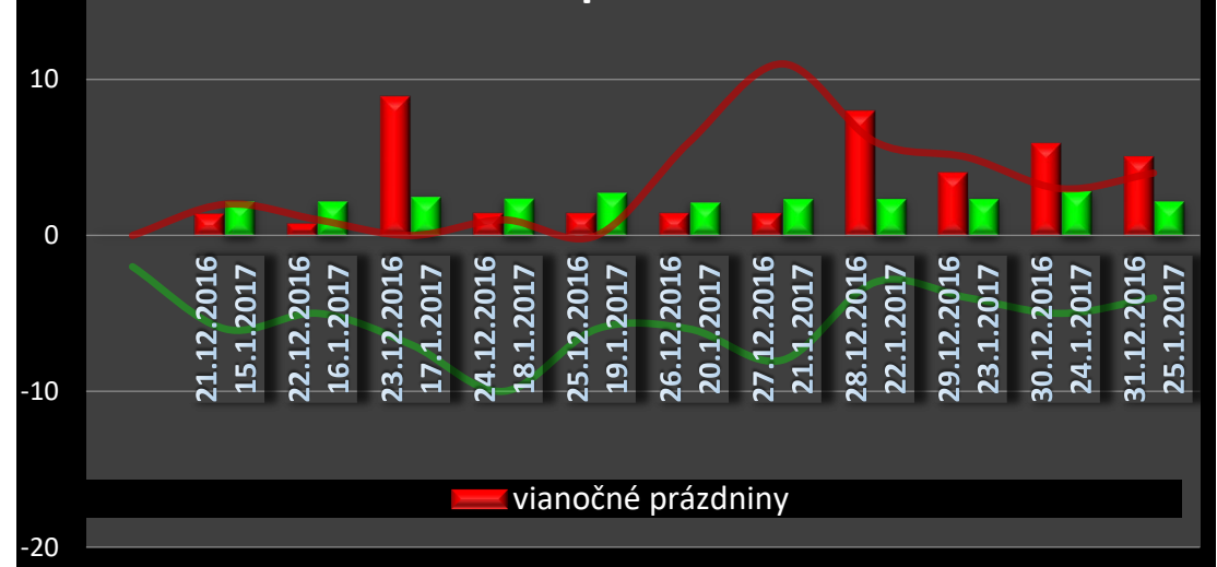
Denné spotreby v MWh k vonkajšej teplote
